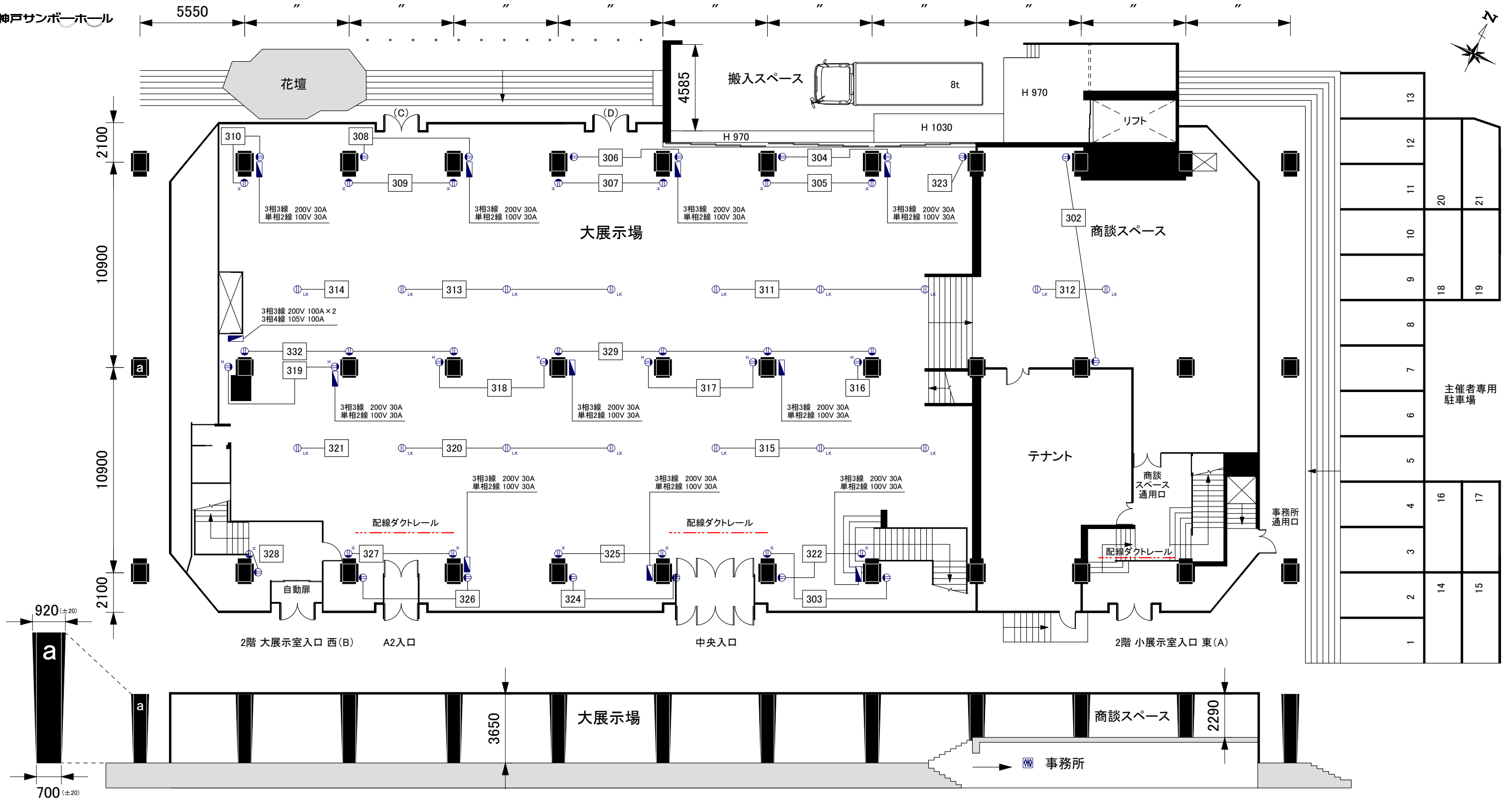
神戸サンボーホール 1階 電気設備図
