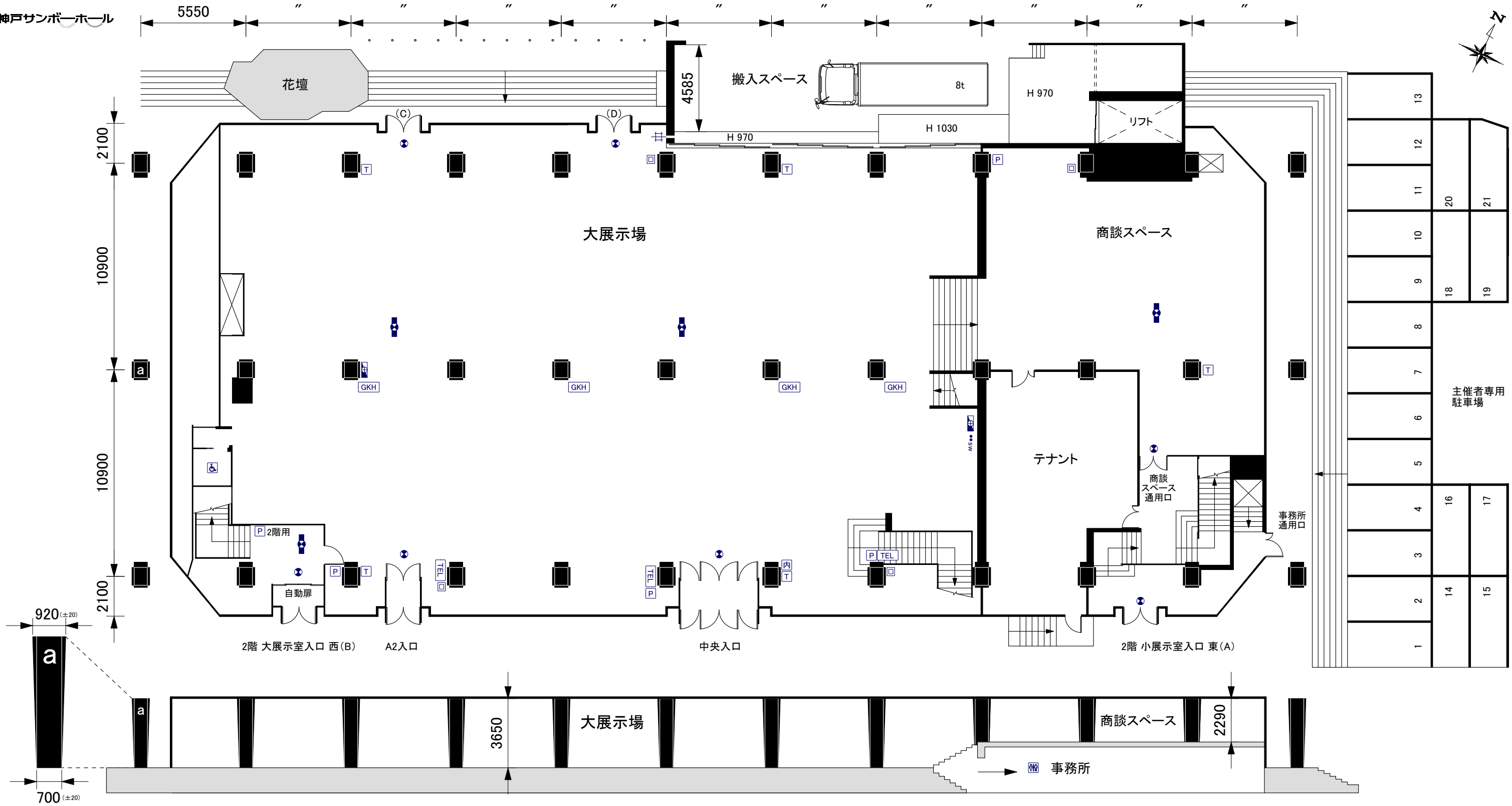
神戸サンボーホール 1階 設備図
