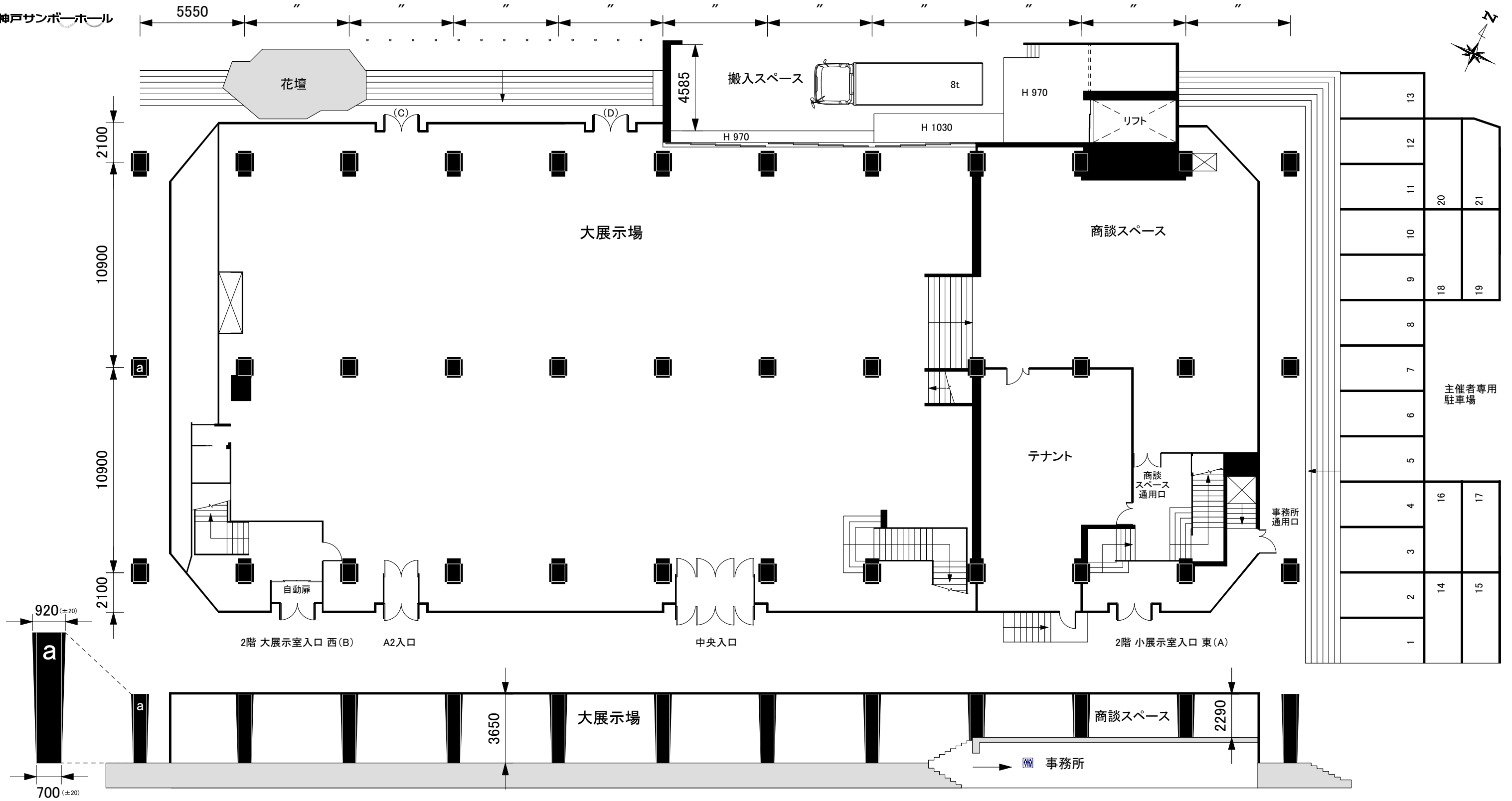
神戸サンボホール 1階 平面・立面図
