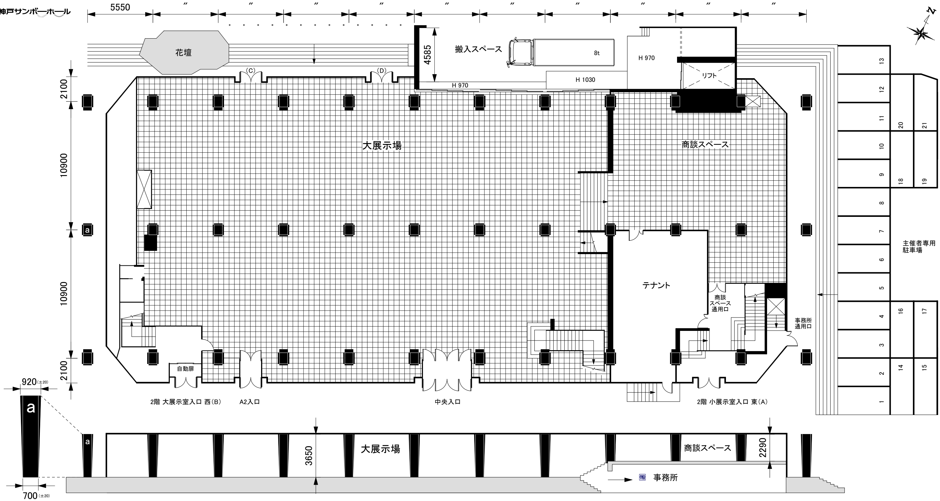
神戸サンボーホール 1階 平面・立面図 タイル目地 (1枚 450×450mm)
