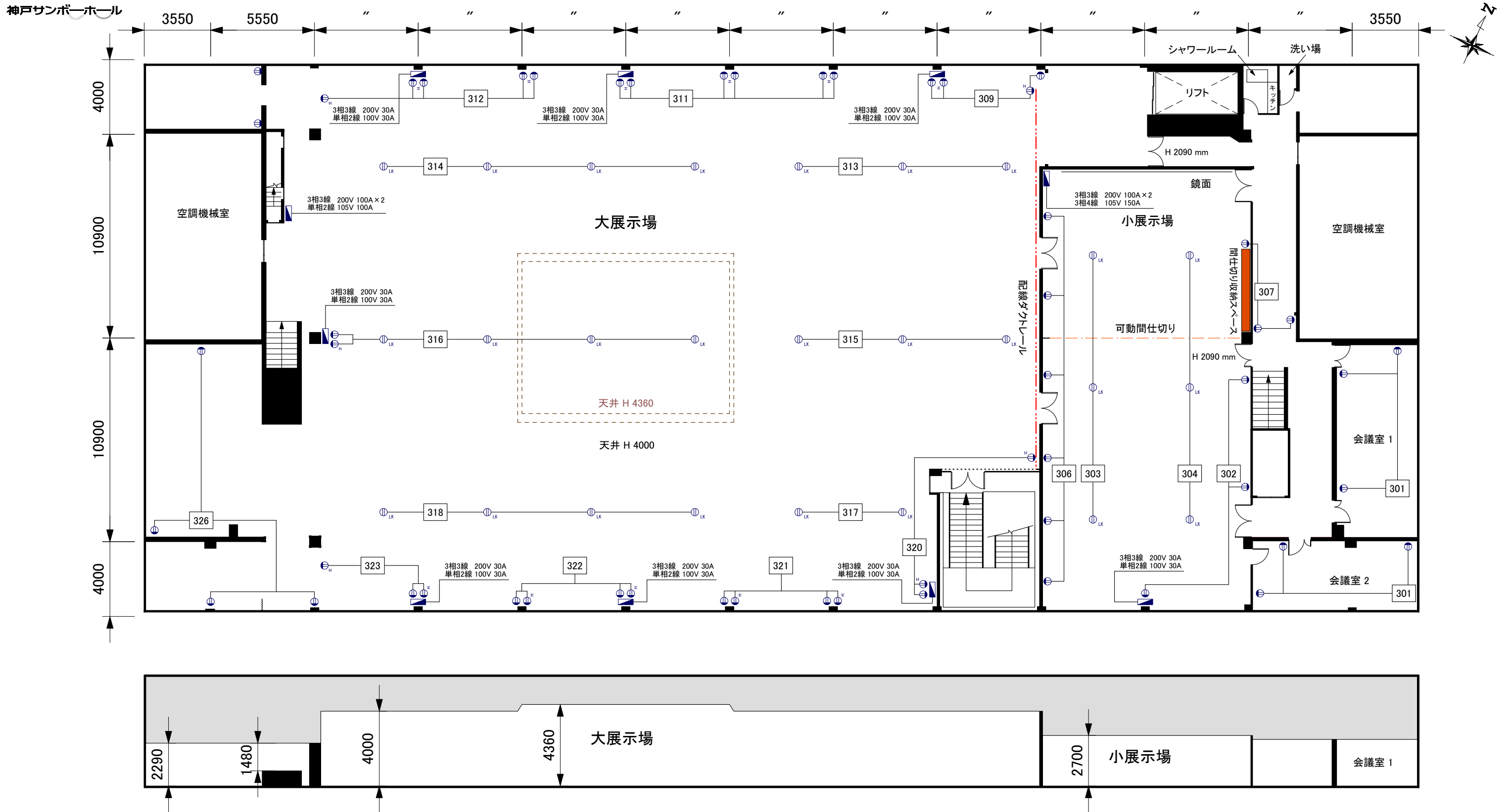
神戸サンボホール 2階 電気設備図
