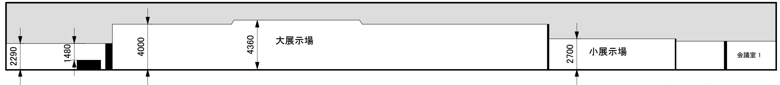
神戸サンボーホール 2階 平面・立面図 タイル目地 (1枚 450×450mm)
